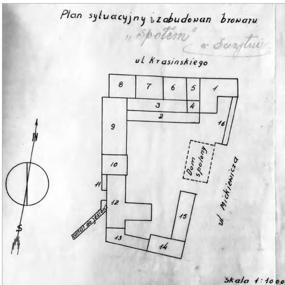
Ryc. 23 – plan sytuacyjny browaru spółdzielni „Spółem” w Szczytnie. Na planie oznaczono: 1 – warzelnia i śrutownik, 2 – hala ekspedycyjna, 3 – rozlewnia piwa butelkowego, 4 – lokal mycia masy filtracyjnej, 5 – kotłownia, 6, 7, 8 – leżakownia, 9 – rozlewnia do beczek i pechownia, 10 – skład lodu, 11 – magazyn beczek, 12 – biura, warsztaty i stołówka, 13 – szopa (magazyn skrzynek na piwo), 14, 15 – garaże, brama i wartownia.
