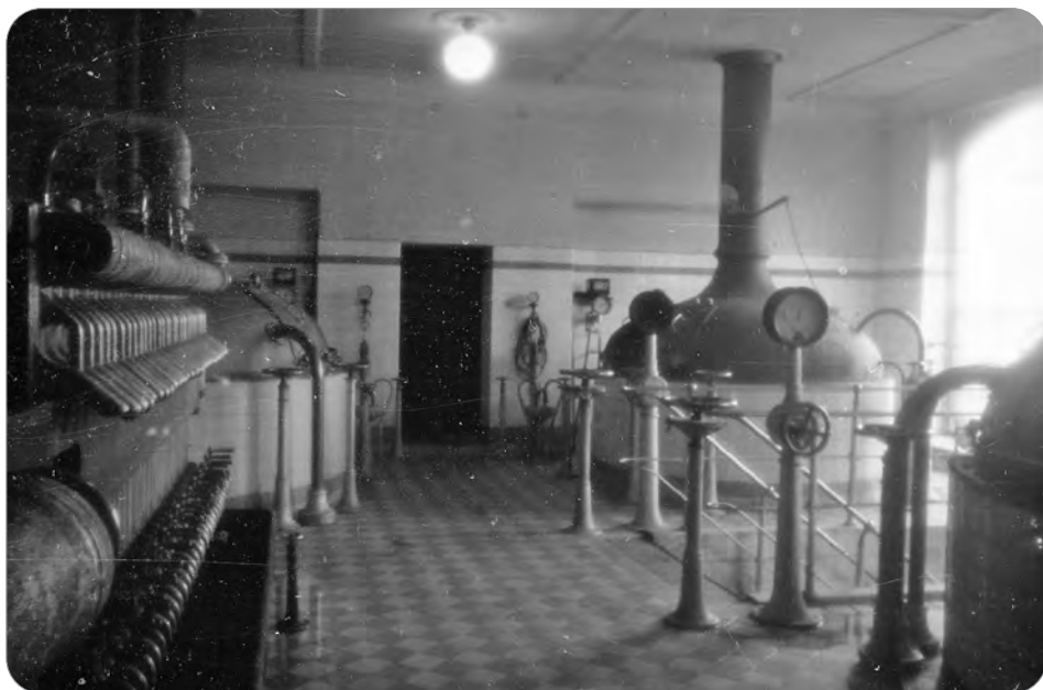
Ryc. 2 – wnętrze warzelni browaru w Polczynie-Zdroju, koniec lat czterdziestych. Po lewej stronie widoczny jest filtr zacierowy (używany zamiast kadzi filtracyjnej). W tle po prawej kocioł warzelny.
