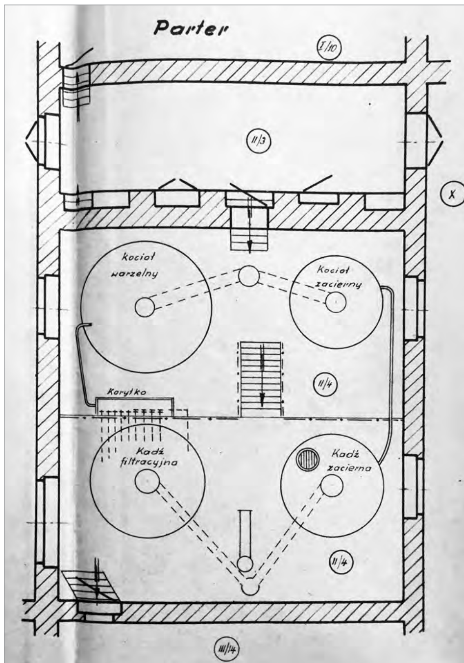
Ryc. 24 – plan warzelni browaru w Zielonej Górze, stan około 1948 roku.
