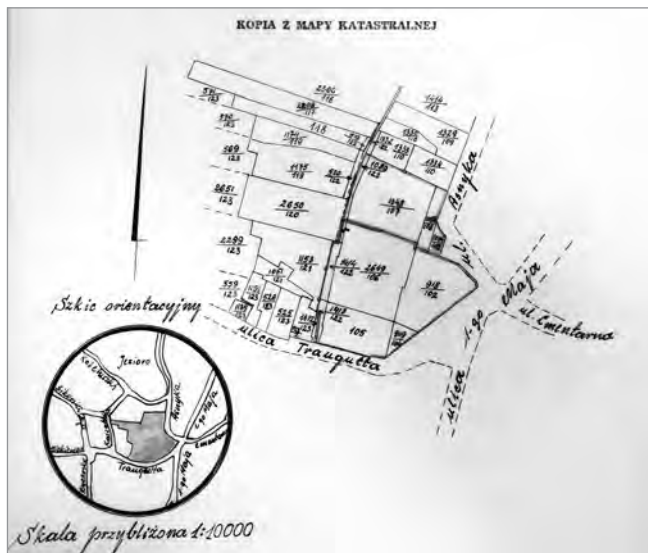
Ryc. 17 – plan usytuowania browaru w Kętrzynie. Lata trzydzieste (na górze). Koniec lat czterdziestych (na dole).
