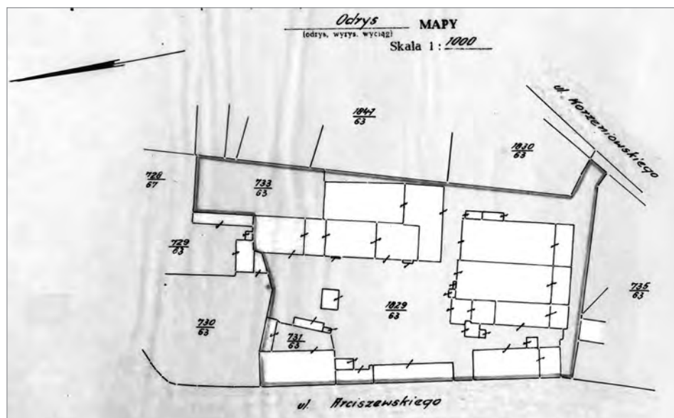
Ryc. 20 – plan sytuacyjny browaru w Nowej Soli (ul. Arciszewskiego 8), koniec lat czterdziestych.
