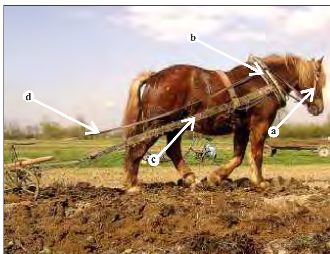
Groty 2 – CzG, Łp, NB, Rp [groty kónskie – Nd; rzond – Fr; uprzong – Dr; uprzonz – Rp]; fot. AJ a – huzda – CzG, Fr [uzda – Fr] b – chomont z PODKŁADEM c – pas – Dr, Fr [pobocek – Fr, Fs, Jw, Kc, Kr, ŁN, Łp, Rp; pobocnik – Łp] d – lyce – ogsp.
