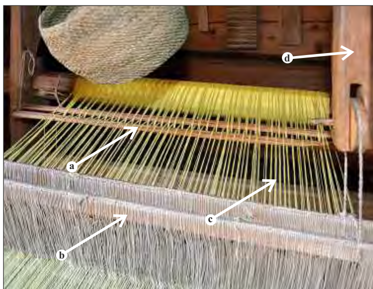
Synka 1 – CzG, Jw, Nd [bic – Fr, Fs, ŁN, Nd, Tr]; fot. KrK; ze zbiorów MT-CzG a – synka b – nicielnice c – osnowa d – lalka
