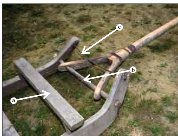
Gnatki 1; fot. JK a – nosod b – wolek c – spinac
