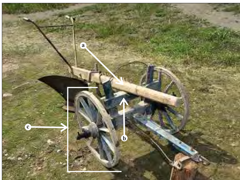
Grzondziyl – CzG, Fr, Fs, Jw, Kc, ŁN, Łp, Rp [gronzel – Fr, ŁN, NB; gronziel – Nd; gronziyl – Fr, ŁN; gróndziel – CzG; grónzel – CzG, Fr, Kr, ŁN, Nd, Tr; grzonziel – Nd; grzónziyl – Fr, ŁN, Nd]; fot. JK a – grzondziyl b – jarzmecko – CzG, Nd [jarzmica – CzG] c – kolca – CzG, Fr, Fs, Jw, Nd [kolce – Jw, Kr, Nd, Tr]
