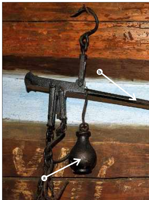
Gruska 5 w WIYNCIYRZU – Nd; fot. JK ze zbiorów MuzPodh a – gruska b – belka
