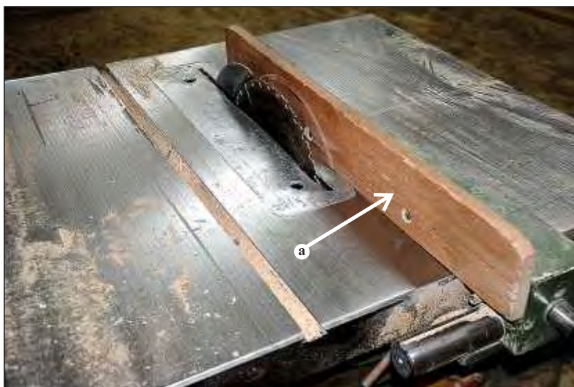
Cyrkulorka – Fr, ŁN, Nd [cylkularka – Kc; cylkulorka – Nd, Tr; cyrkula – Jw] fot. JK a – culaga – Kc
