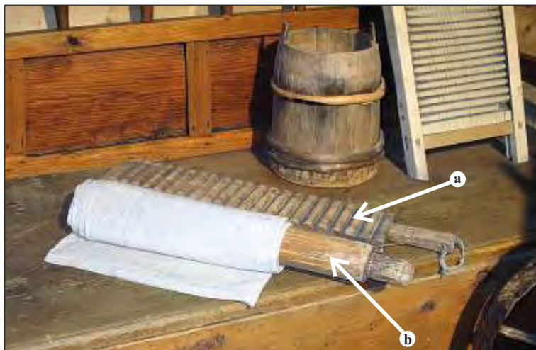
Kijonka 2 – CzG, Fr, Kc [garbula – Rp; kijonka garbato – CzG, Jw, Łp, Rp; rajbacka]; fot. KrK; ze zbiorów MT-Jurg a – kijonka b – tocko – CzG, Fr, Fs, Jw, Kc, ŁN, Nd, Rp
