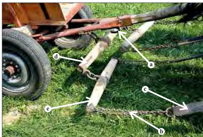
Fornogiel – Fr, ŁN, ŁW, Nd [ hok – ŁW ]; fot. JK a – fornogiel b – nokóniec – NB [ górcik – Nd; kóncówka – CzG, Łp, Rp; postrónek – Fr ] c – pas – Dr, Fr [ pobocek – Fr, Fs, Jw, Kc, Kr, ŁN, Łp, Rp; pobocnik – Łp ] d – woga – Fr, Fs, Tr e – orcyk – ogosp. [ barco – Fr; horcyk – Fr; worcyk – Kc, Tr ]
