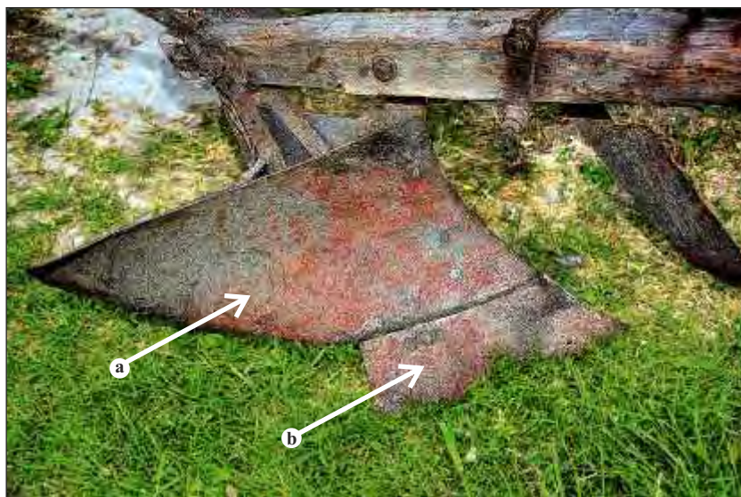
Odwalnica – Fr, Tr [blacha – ogsp.; deska – Fr; isty – Kr, Łp; odkładnica – Fr, Fs, Nd, Rp, Tr; skrzidło – Kr, Łp] fol. JK a – odwalnica b – lymiys – ogsp. [lymies – Fr; nałózka – CzG, Jw; nokłod – Fs, Kc, ŁN, Łp, ŁW, Nd, Tr; nokłodka – Dr, Fr, Jw, Kr, NB, Nd, Tr; nołózka – CzG]
