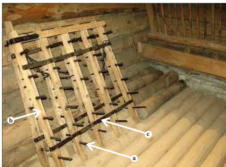
Brona 1 – ogsp. [bróna – CzG, Fr, Jw, ŁN]; fot. KrK a – bronik – ogsp. [brónik – Fr, Jw] b – słupek – CzG c – syda – Fr, Fs
