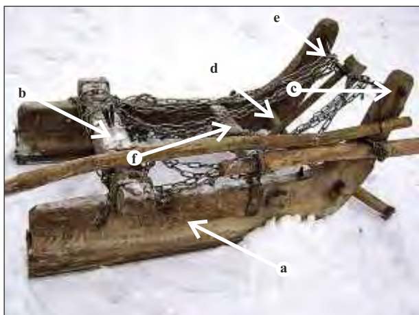
Gnatki 2 – model w MEK – ogsp. fot. JK; ze zbiorów ME w Krakowie
