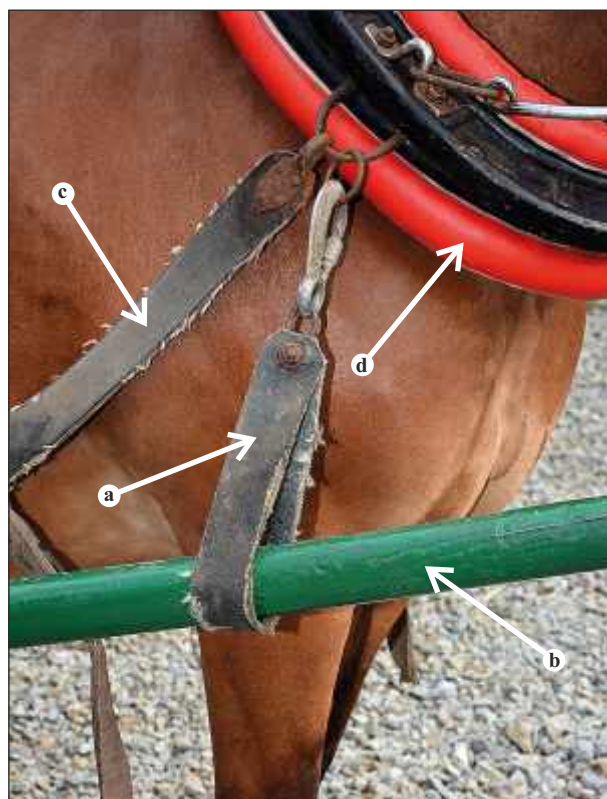
Biegunka 2 – Rp; fot. JK
