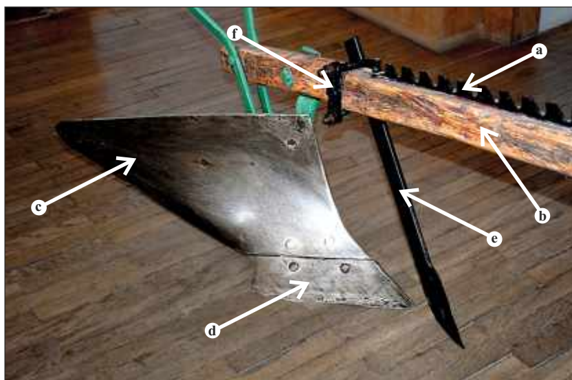
Grzebiyń 2 – Fr [piylka – Kr; zymbówka – ŁW]; fot. JK a – grzebiyń b – grzondziyl c – odwalnica – Fr, Tr [blacha – ogsp.; deska – Fr; istyk – Kr, Łp; odkładnica – Fr, Fs, Nd, Rp, Tr; skrzidło – Kr, Łp] d – lymiyś – ogsp. [lymies – Fr; nalózka – CzG, Jw; nokłód – Fs, Kc, ŁN, Łp, ŁW, Nd, Tr; nokłodka – Dr, Fr, Jw, Kr, NB, Nd, Tr; nolózka – CzG] e – trzósło – ogsp. [ciosło – Jw] f – skrynt I 2 – Tr
