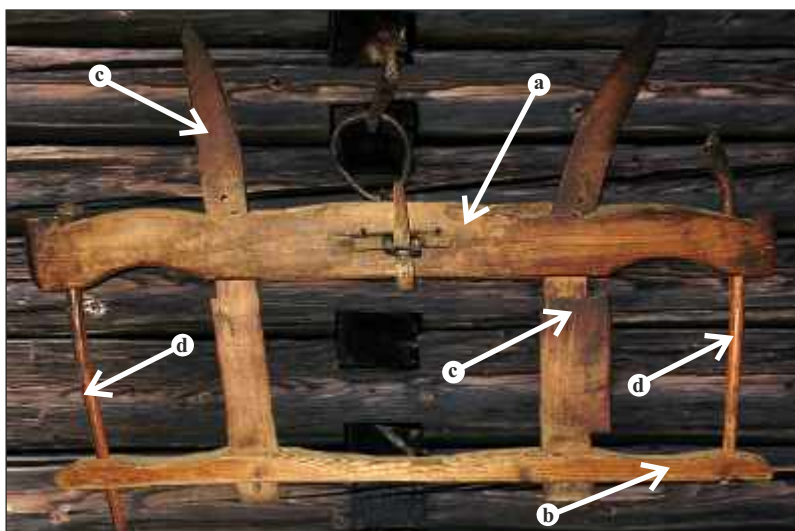
Jarzmo 1 ; fot. JK
